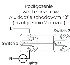
Schemat instalacji łącznika uniwersalnego schodowego.
