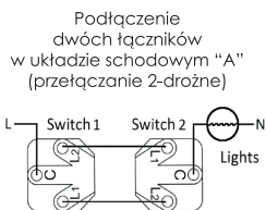
Schemat instalacji łącznika uniwersalnego schodowego.
