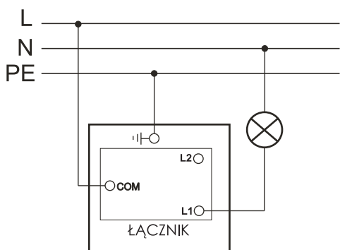
Schemat instalacji łącznika uniwersalnego schodowego.
